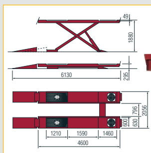
RAV 602 - kg 4000 RAV 642 - kg 5000
