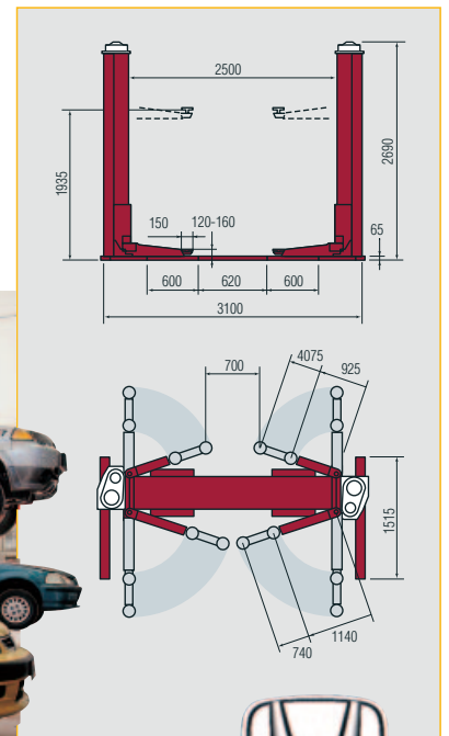
KPS 305 H - kg 2700 KPS 306 H - kg 3200
