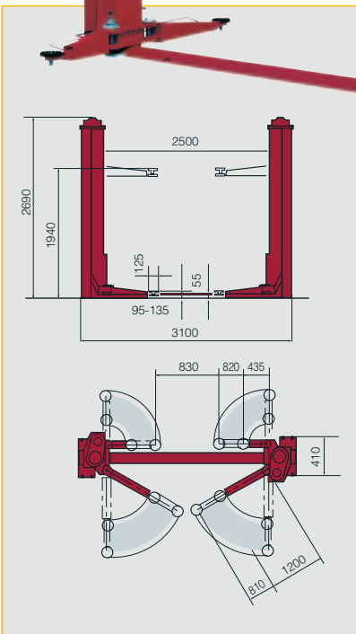
KPS 326 H - kg 2700 KPS 327 H - kg 3200
