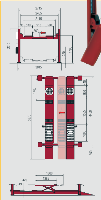
RAV 4212 SI - kg 3500 RAV 4212 NSI - kg 4000
